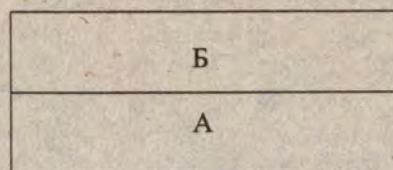
Рис. 1. Природа как компонент натурсоциозкосистемы: две формы бытия природы. А – естественная (неочеловеченная) природа; Б – очеловеченная природа.
