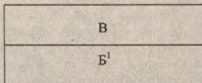
Рис. 2. Общество как компонент натурсоциозкосистемы: два уровня общественной жизни. V – специфический, социальный уровень; B 1 – технологический (природный подчиненный) уровень: очеловеченная природа, рассматриваемая в качестве подчиненного социальному уровню компонента общественной жизни.
